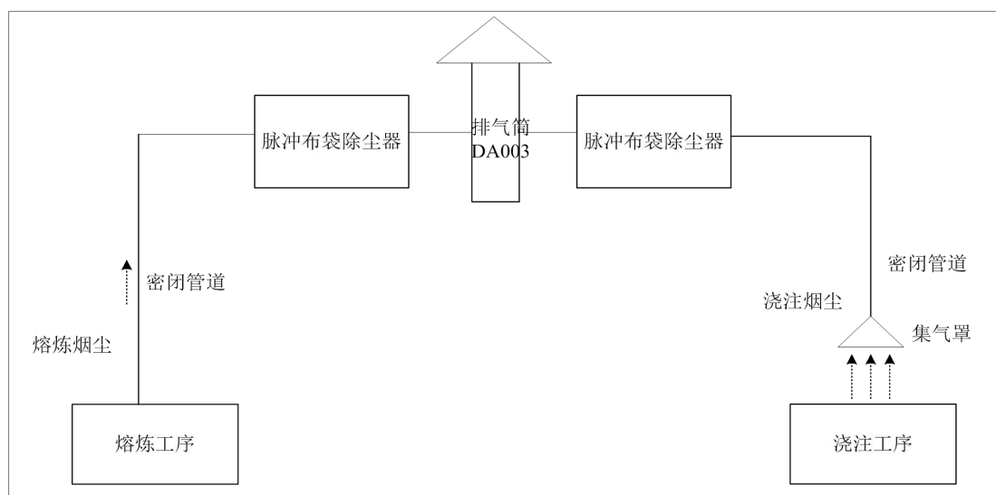
图 4.1-2 废气收集管线示意图（DA003 排气筒）
