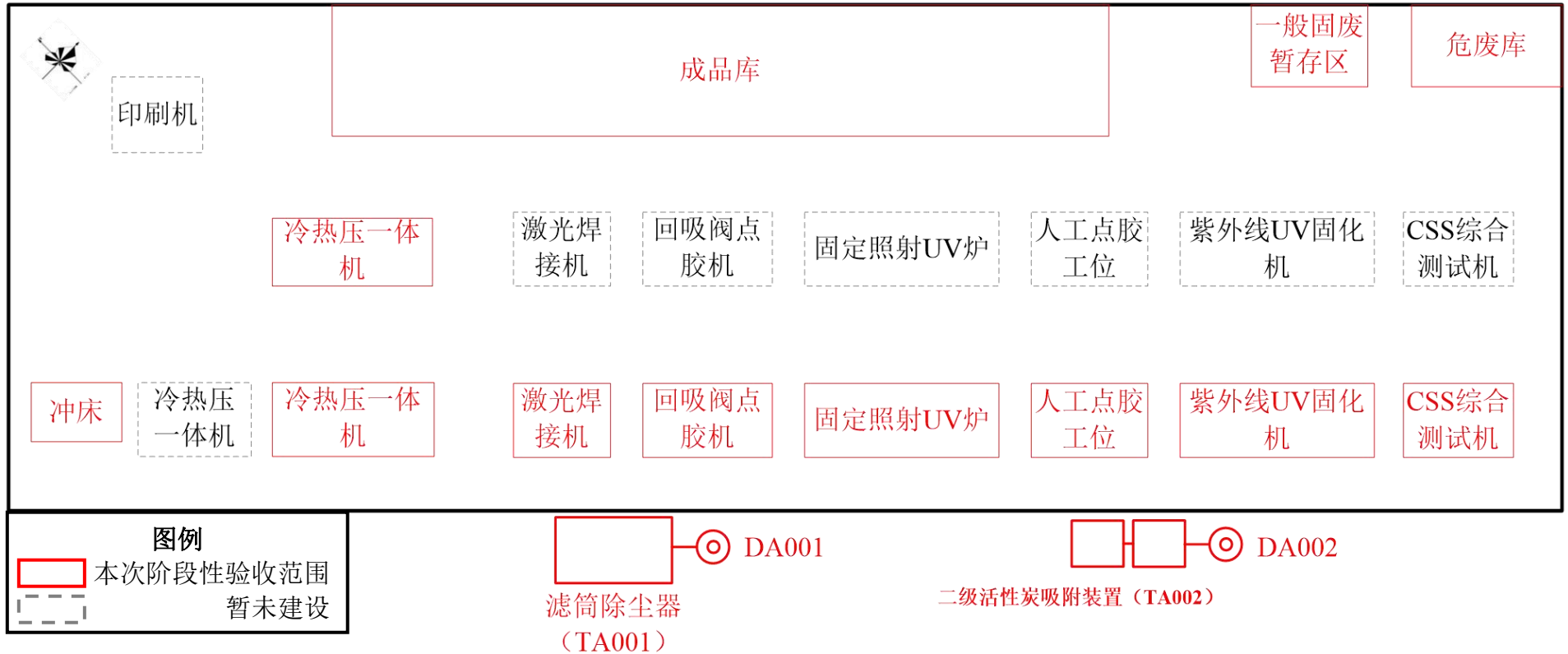
附图 3.1-3 厂房 1 层平面布置图
