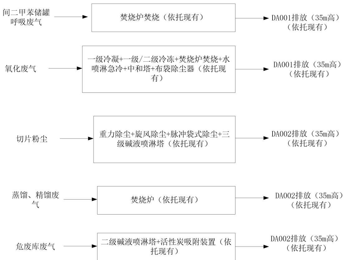
图 4.1-7 废气处理工艺流程图
