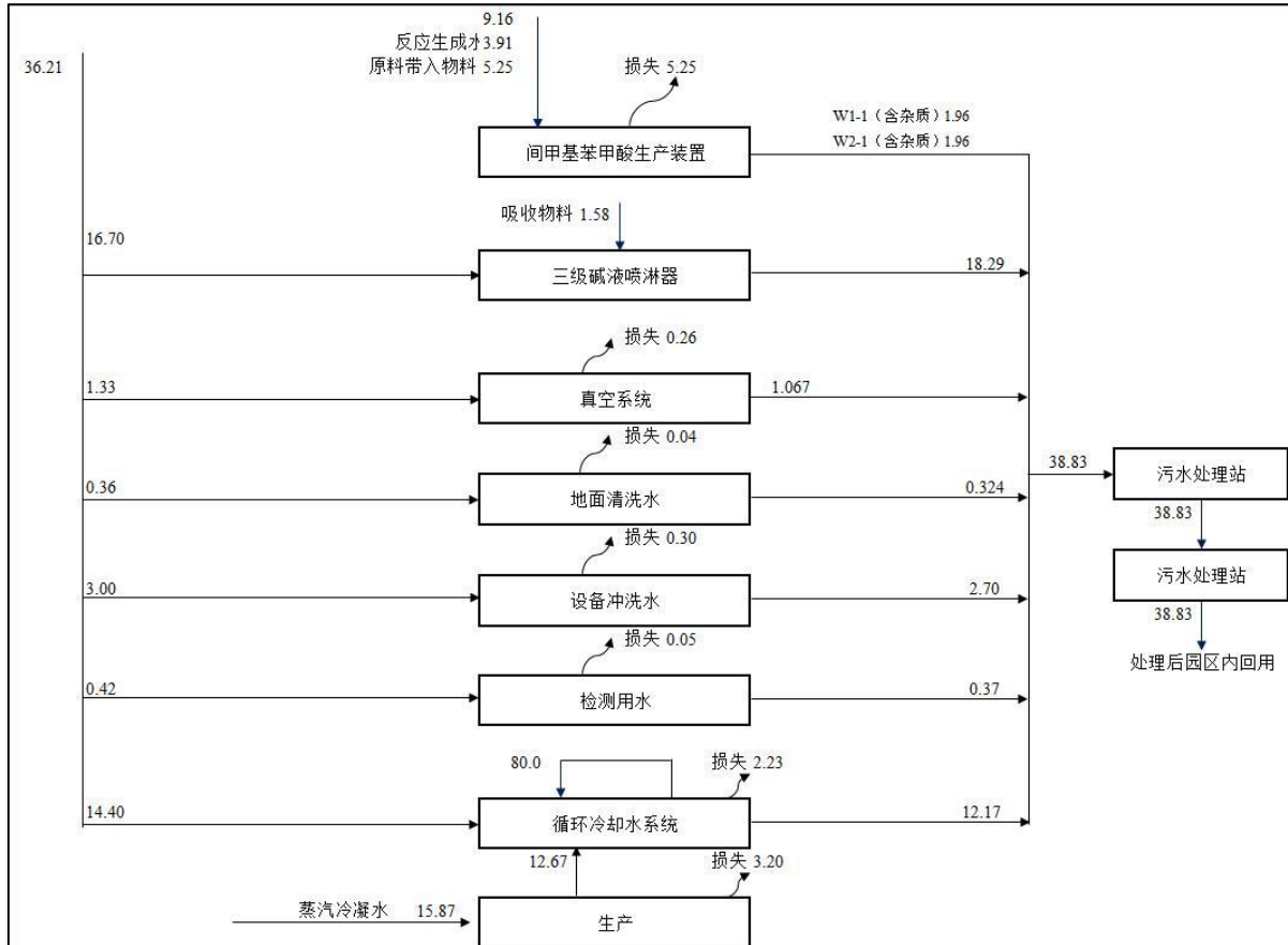
图 3.5-1 本项目水平衡图 (单位: t/d)
